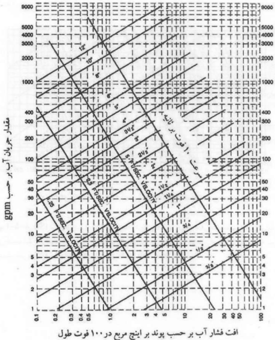
شکل پ ۱-۵-۷ (IP) منحنی اندازه‌گذاری لوله‌های مسی نوع M از استاندارد ASTM B 88
