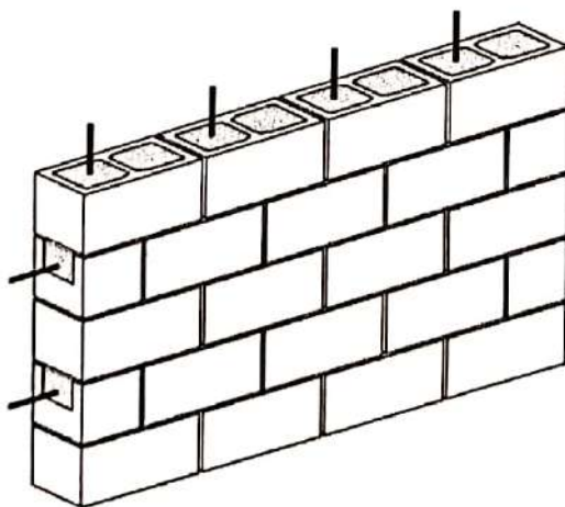
شکل ۱-۴-۸ نمونه‌هایی از دیوار بنایی مسلح
